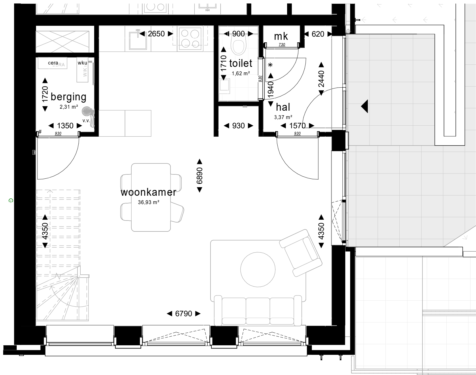
1e verdieping
