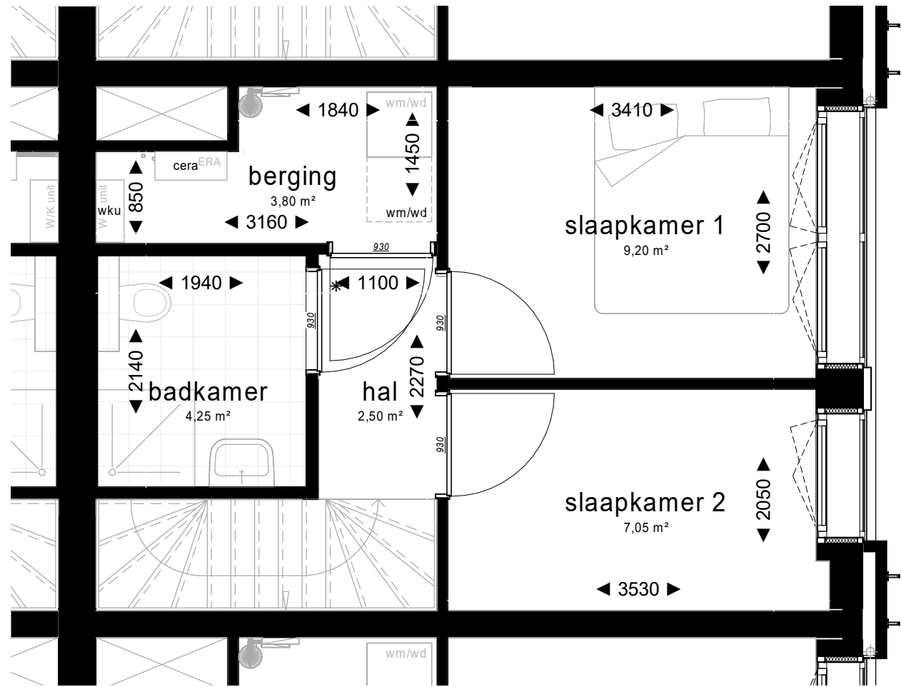
2e verdieping
