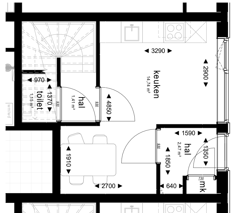
1e verdieping
