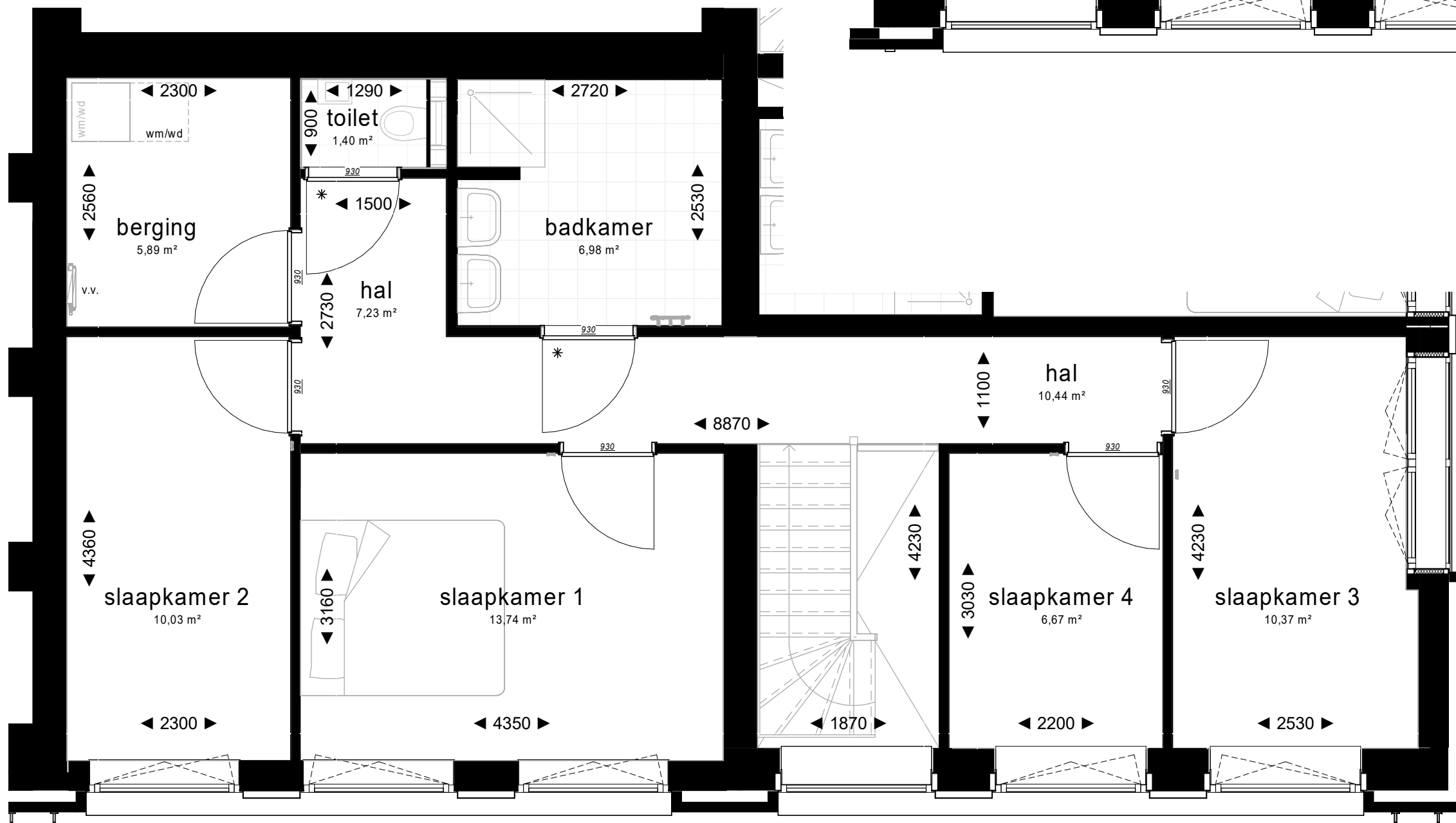
2e verdieping
