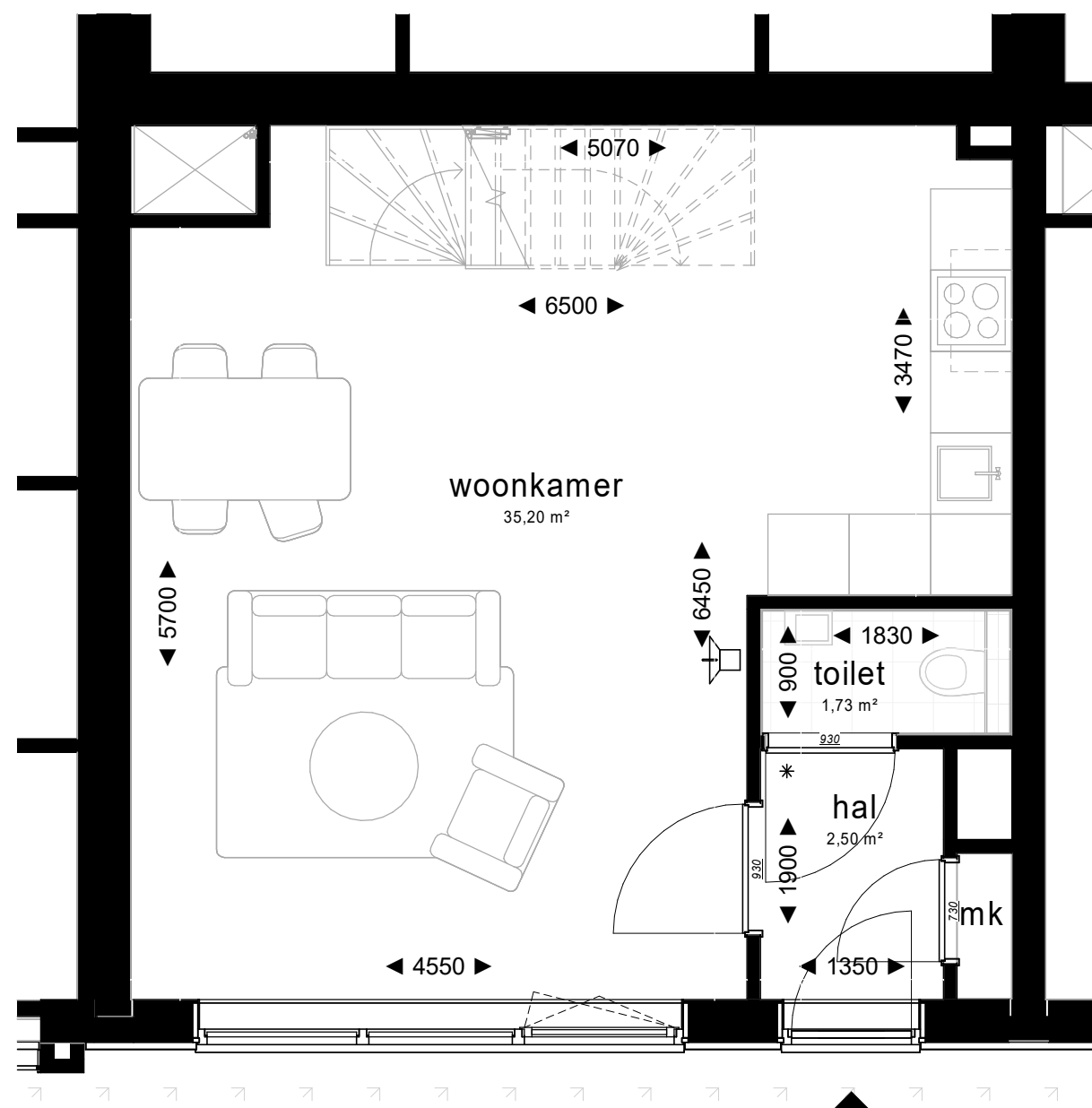
1e verdieping
