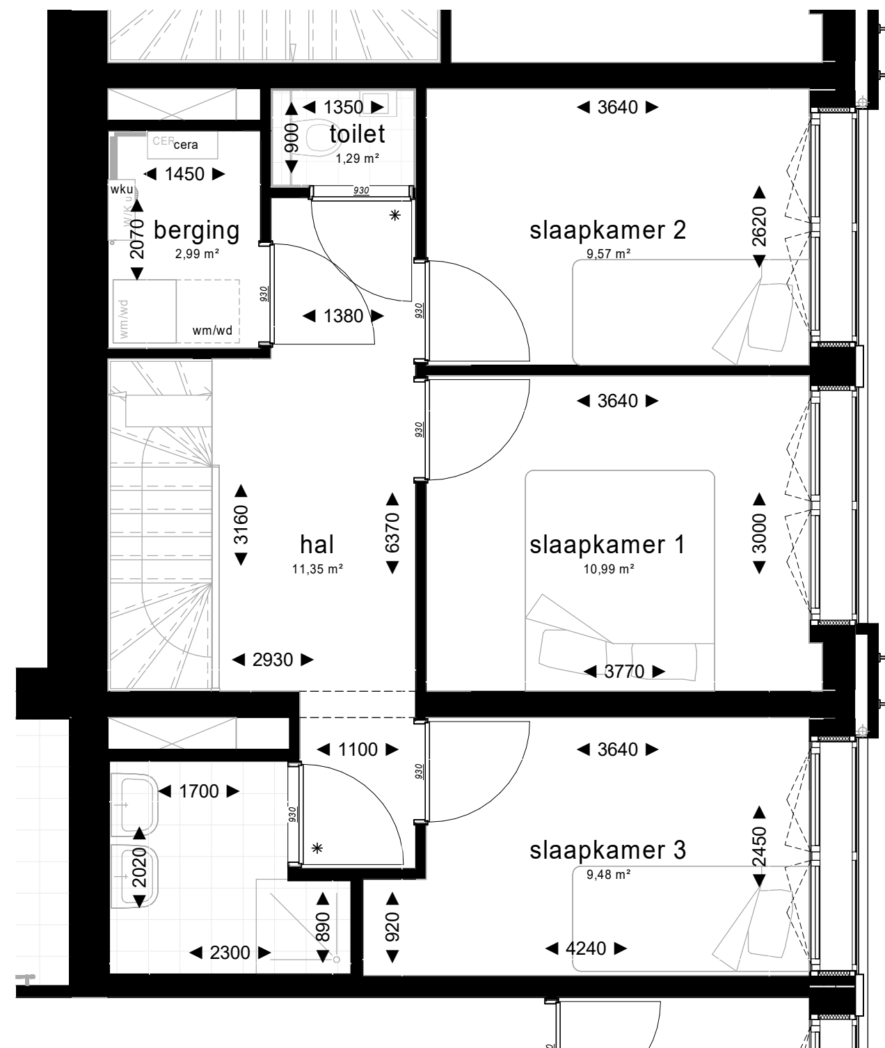
2e verdieping
