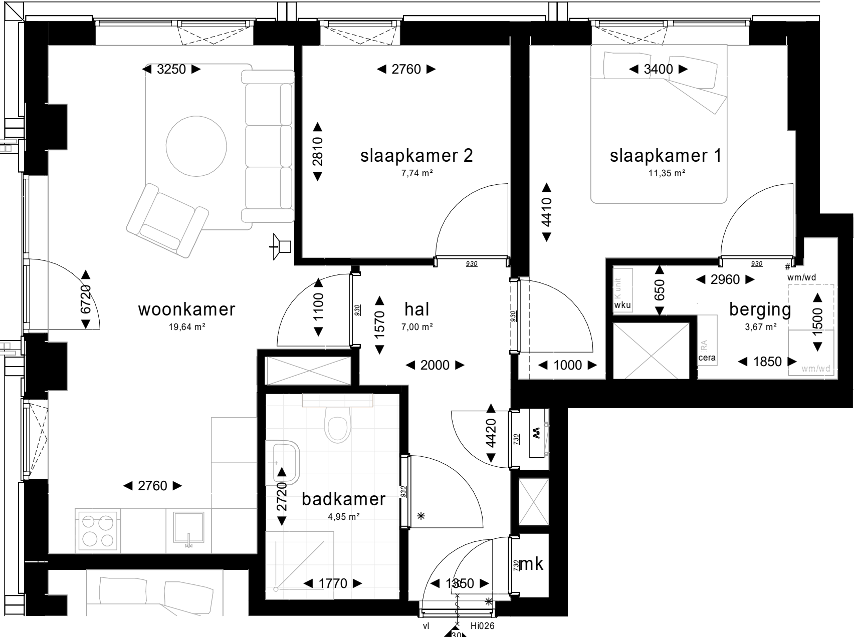
9e t/m 13e verdieping
