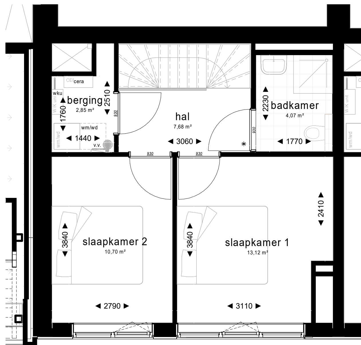
2e verdieping
