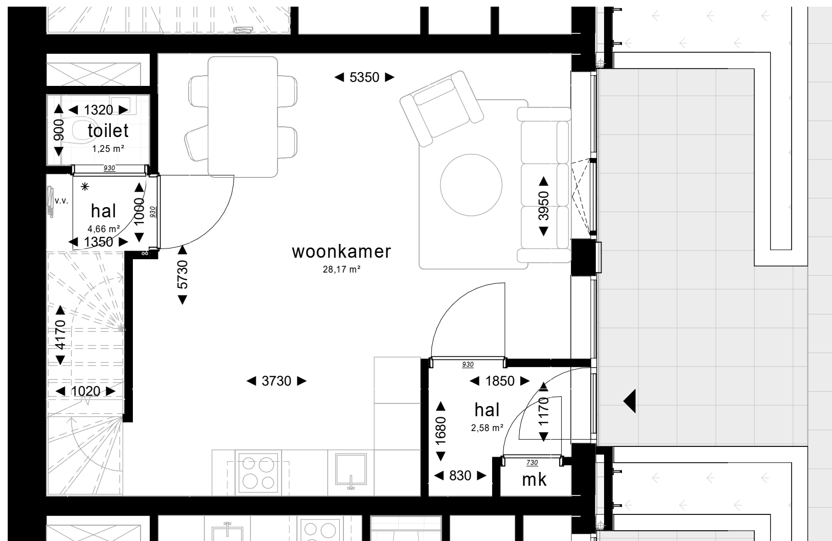
1e verdieping
