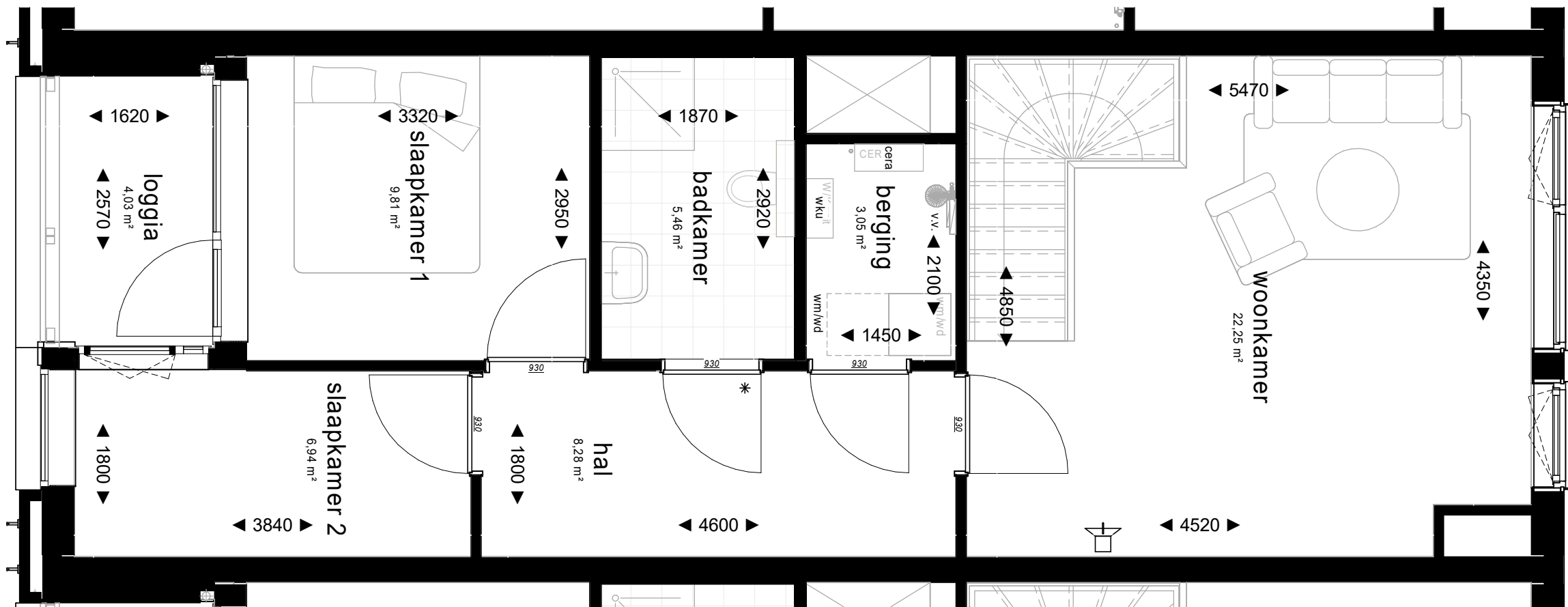
2e verdieping
