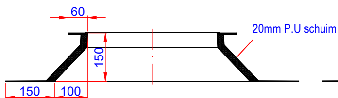
Doorsnede
