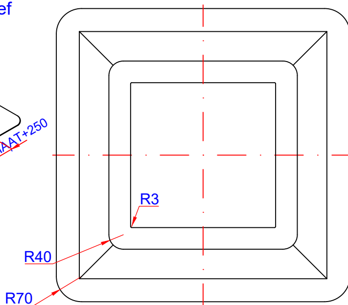
Boven aanzicht
