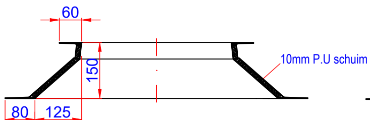
Doorsnede
