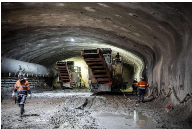
Construction en cours des tunnels de la phase 1 de l'autoroute M6 - Copyright : Transport for NSW
